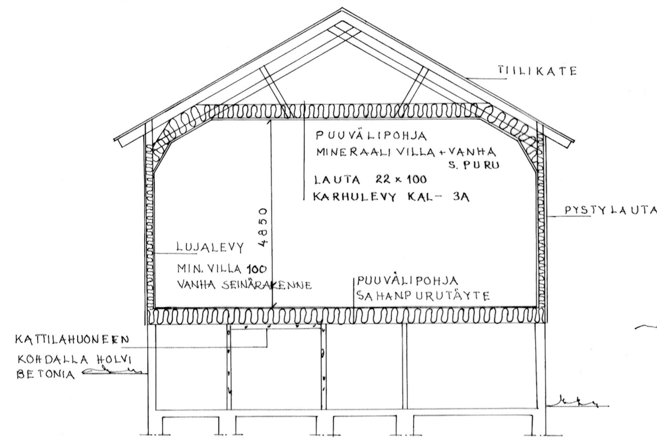
LEIKKAUS A - A
