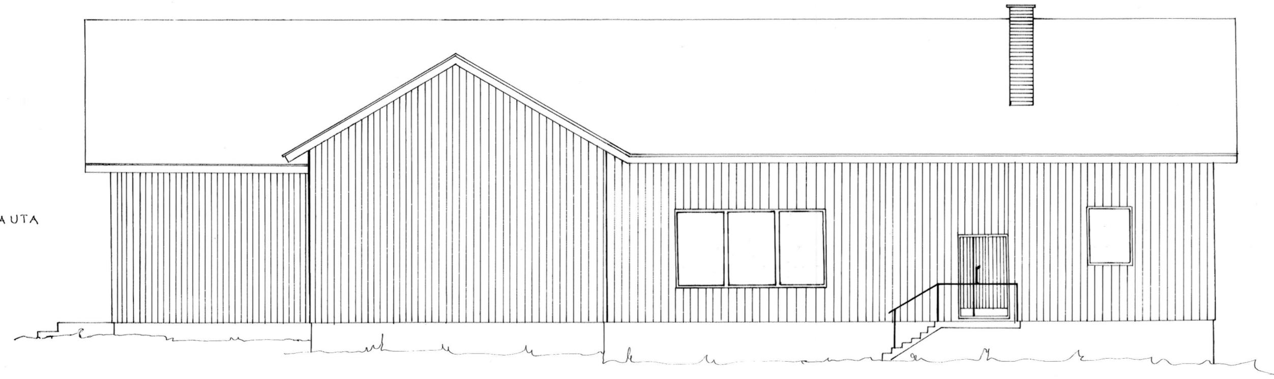
JULKISIVU
