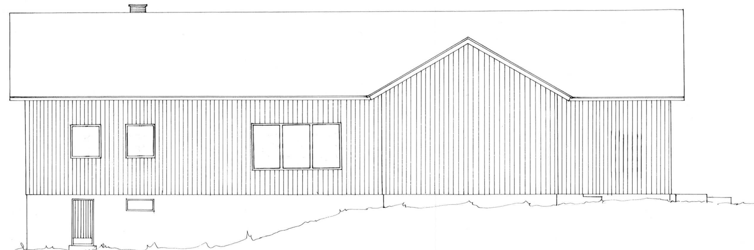
JULKISIVU
