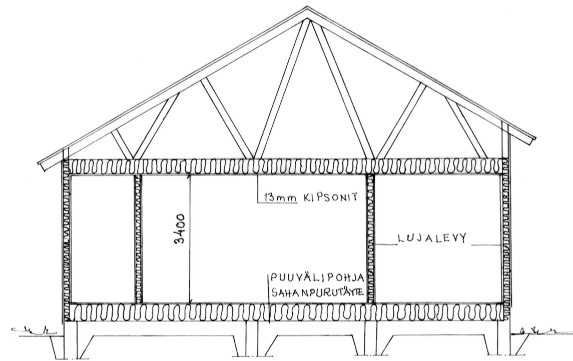
LEIKKAUS B - B
